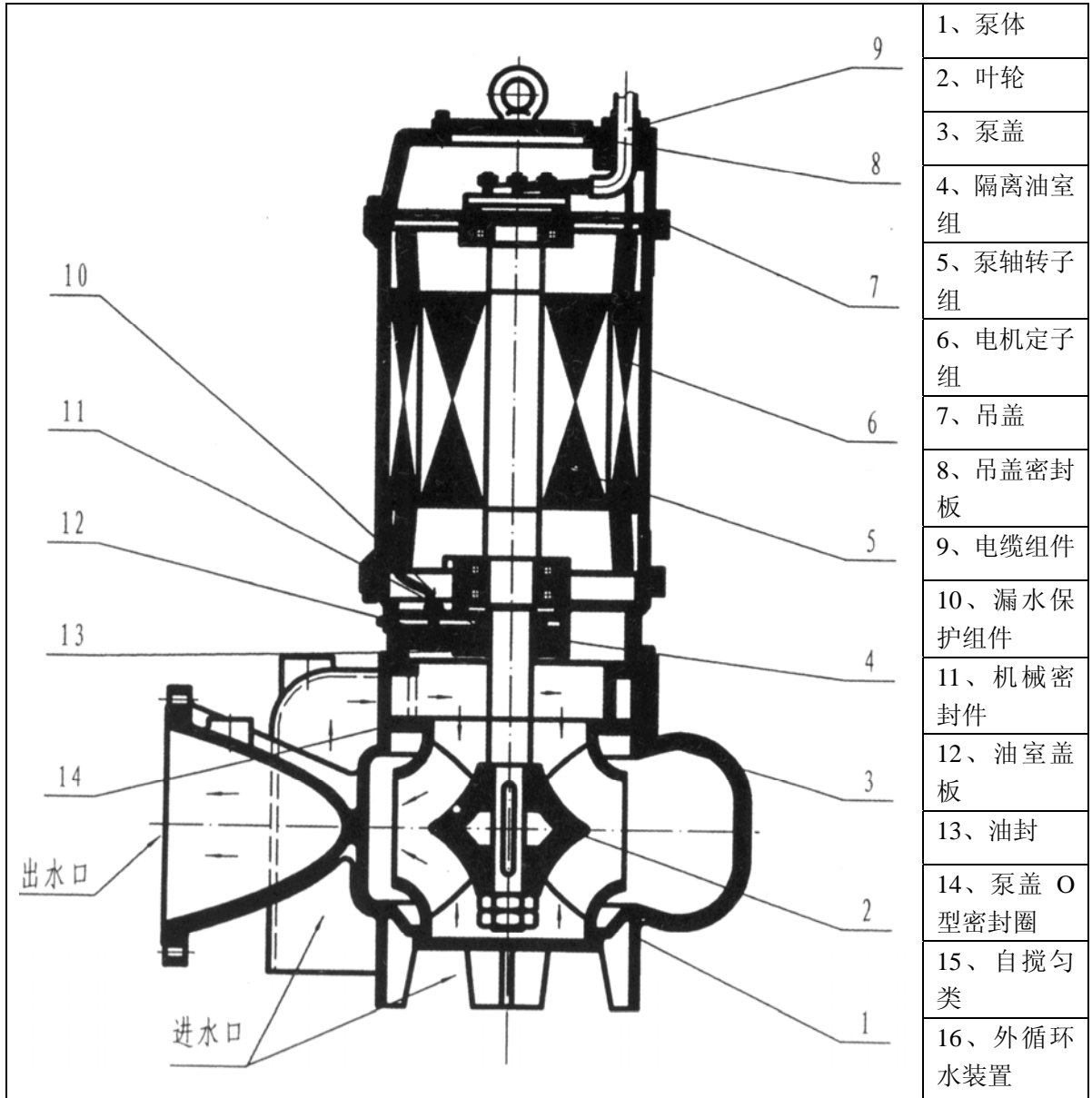
WQS 双吸潜水排污泵结构说明
